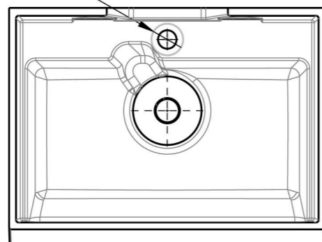
Bottom view/ Widok od dołu \phi 60 Flat area/ Powierzchnia płaska
